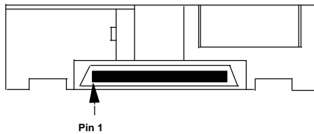
Elektrische Anschlüsse bei den 80-Pin-SCA-Modellen (Rückansicht)
