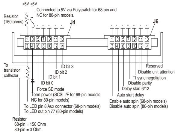
Elektrische Anschlüsse bei den 80-Pin-SCA-Modellen (Rückansicht)
