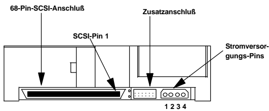
Elektrische Anschlüsse bei den 68-Pin-Modellen (Rückansicht)
